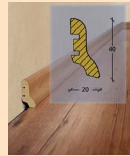
Ktex 4 20 x 40 x 2400 mm
