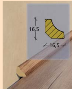
Ktex 3 16,5 x 16,5 x 2400 mm
