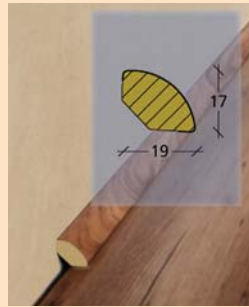
Ktex 2 19 x 17 x 2400 mm
