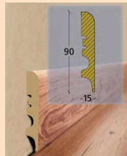
Ktex 7 15 x 90 x 2400 mm
