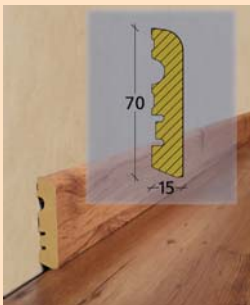
Ktex 5 15 x 70 x 2400 mm
