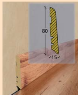
Ktex 6 15 x 80 x 2400 mm
